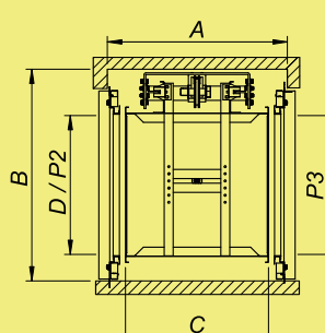
DOBLE EMBARQUE 180°
