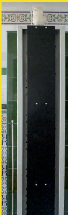
Impulsión por medio de cilindro hidráulico de empuje directo. Guías cerradas en chapa para evitar accidentes.
